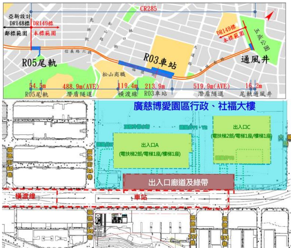
R03站平面位置示意圖
